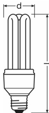
DSST STICK 17 W/825 E27, DSST STICK 17 W/840 E27
