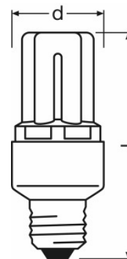
DSST STICK 8 W/825 E27, DSST STICK 8 W/840 E27
